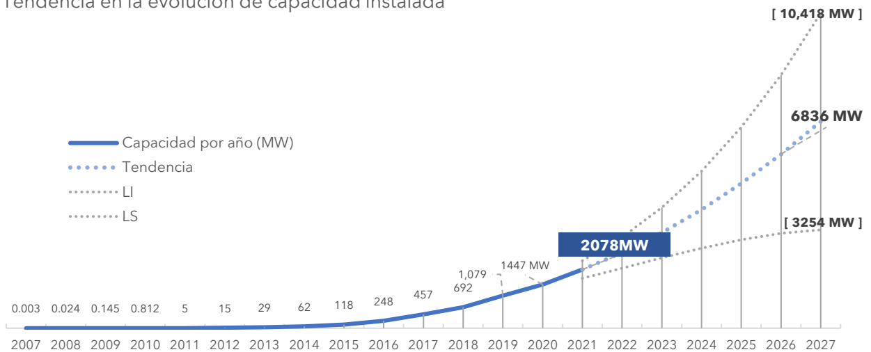
Figura XI.4 Tendencia de la capacidad instalada en Centrales Eléctricas con capacidad menor a 500 kW.
