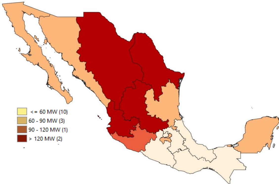
Figura XI.2 Capacidad integrada de Centrales de Generación Distribuida por División de Distribución.
