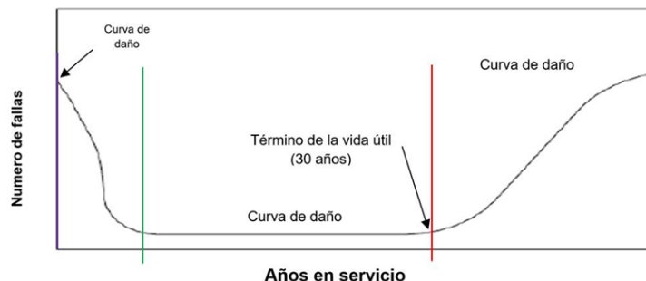
Figura VIII.1 Curva de daño de elementos de transformación de alta a media tensión.
