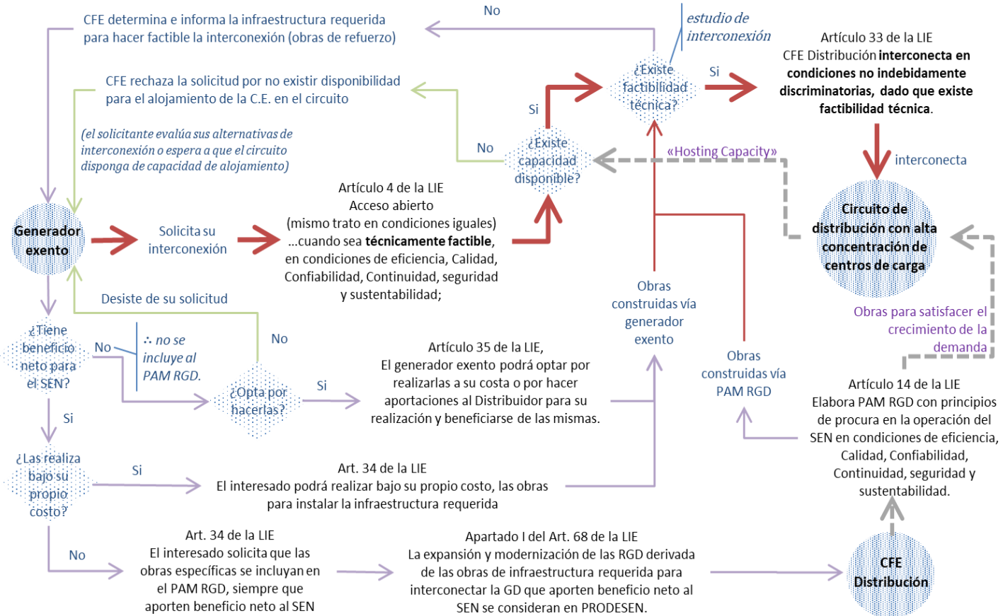
Figura XI.1 Estrategia para considerar en el proceso de planeación de las RGD los requerimientos de ampliación y modernización de la infraestructura eléctrica asociados con el incremento en la Generación Distribuida.
