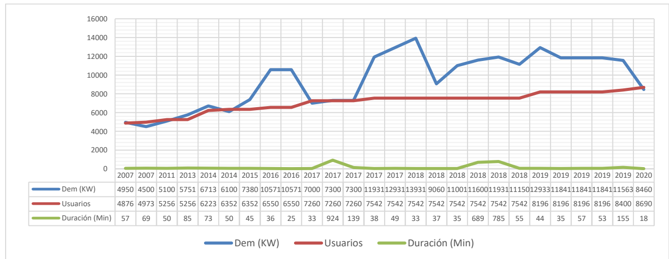
Figura IX.3 Historial de fallas en el cable de energía de Isla Mujeres de 2007 a 2020.
