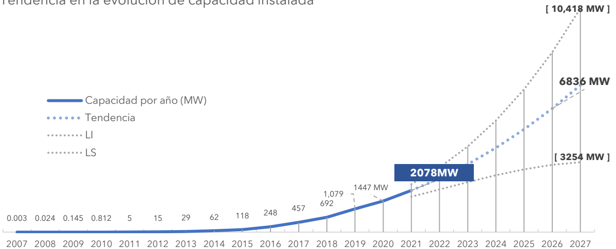
Figura IV.3 Tendencia de la capacidad instalada en pequeña y mediana escala.
