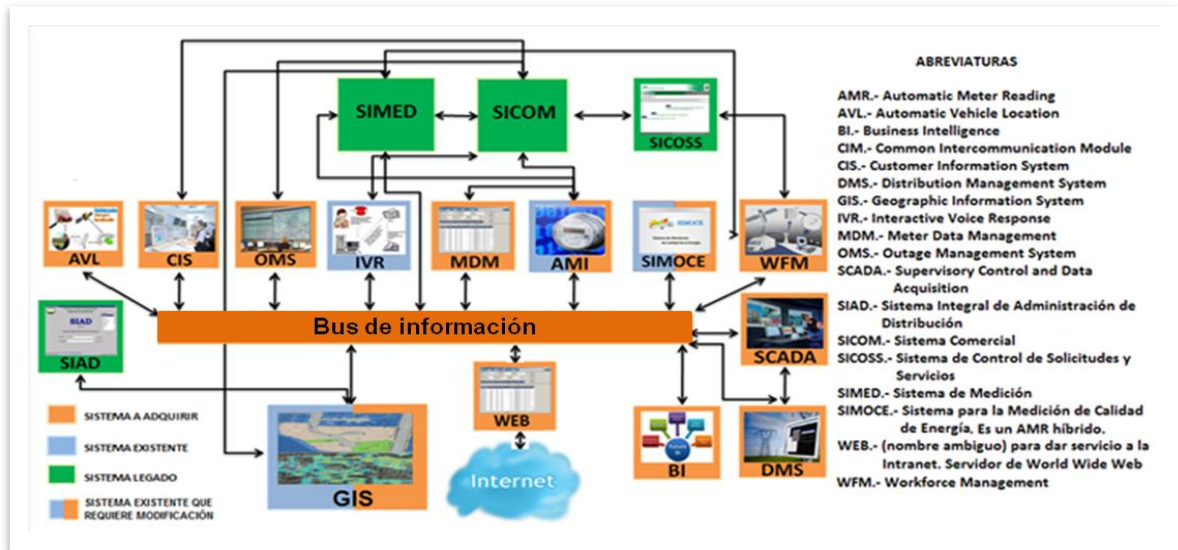
Figura X.1. Principales componentes de una Red Eléctrica Inteligente (REI) en distribución.
