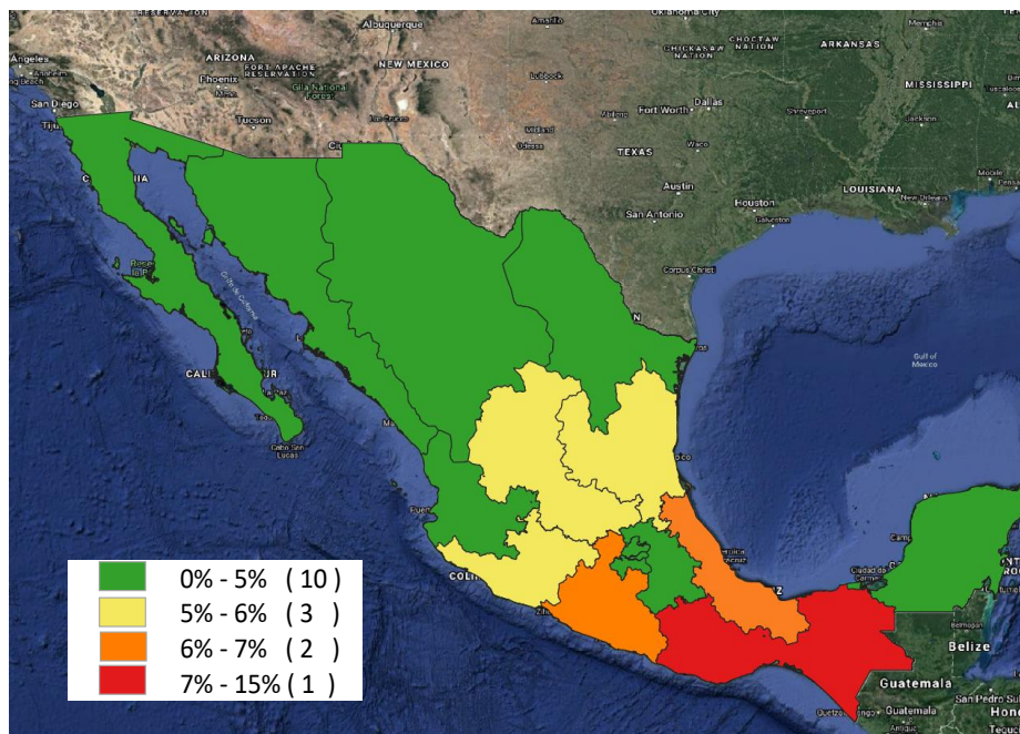
Figura V.9 Mapeo del índice de pérdidas técnicas en Media y Baja tensión por División de Distribución.
