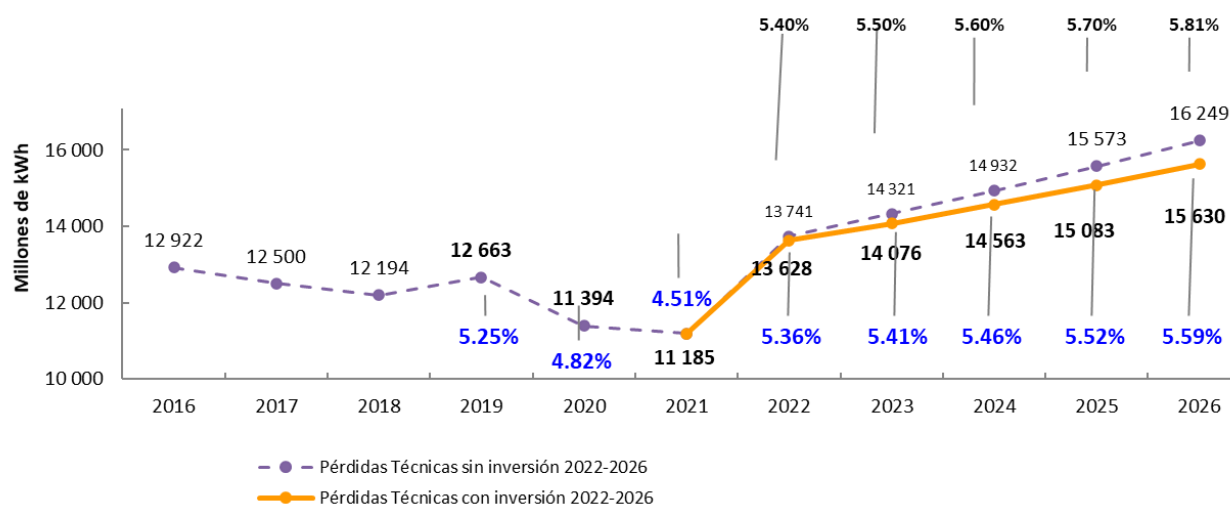
Figura V.10 Proyección de pérdidas de energía con inversión en los años 2016-2021.
