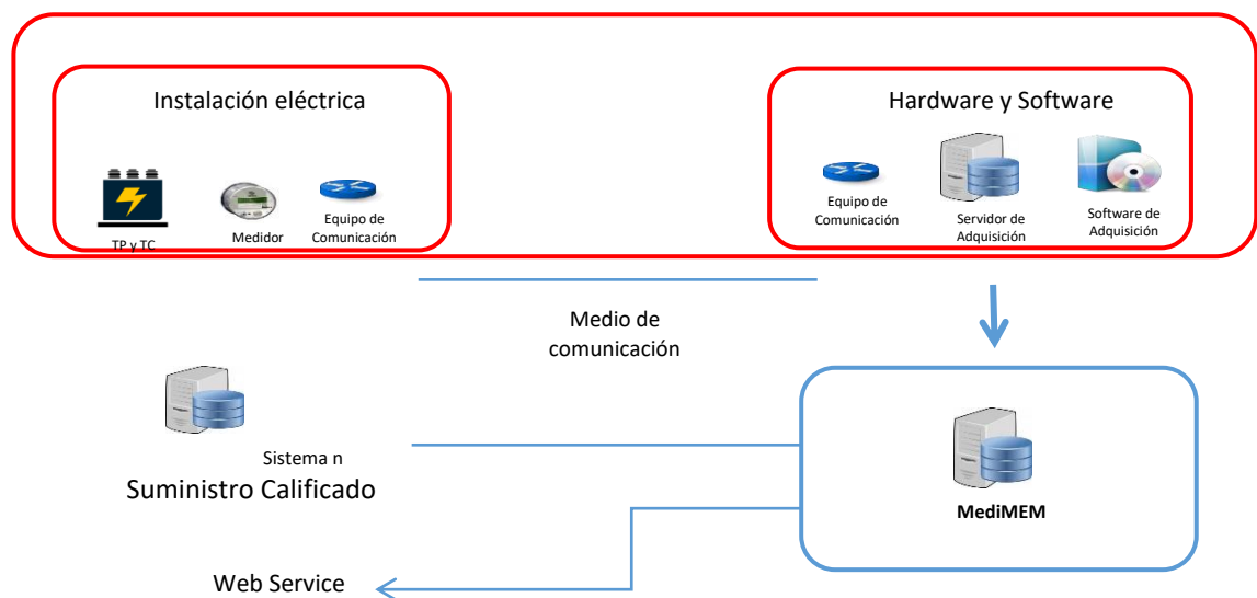
Figura X.4. Esquema general de equipos, componentes e interconexión para los puntos de medición al exterior de subestaciones
