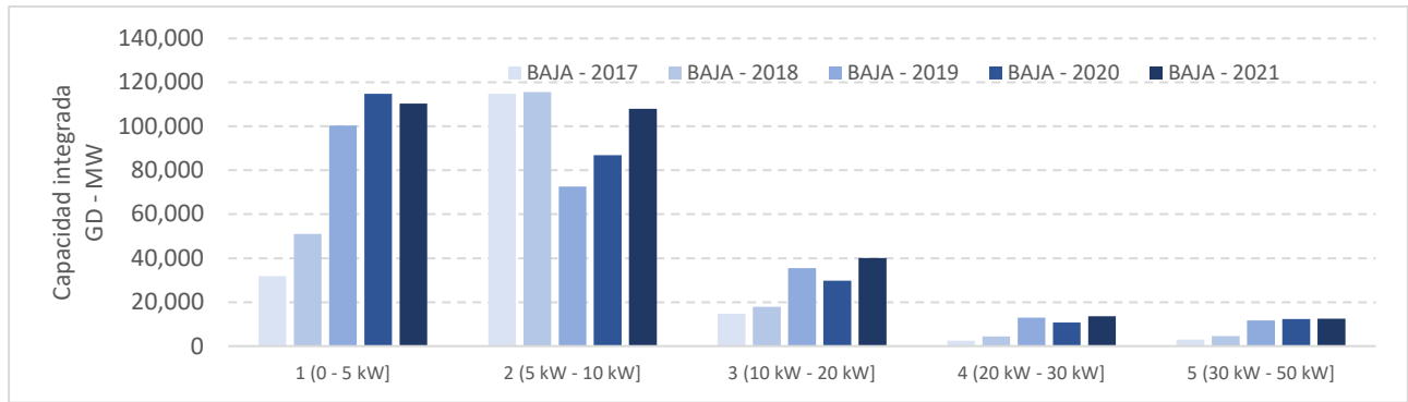
Figura XI.7 Evolución de la capacidad de generación integrada a las RGD anualmente en baja tensión, de 2017 a 2021
